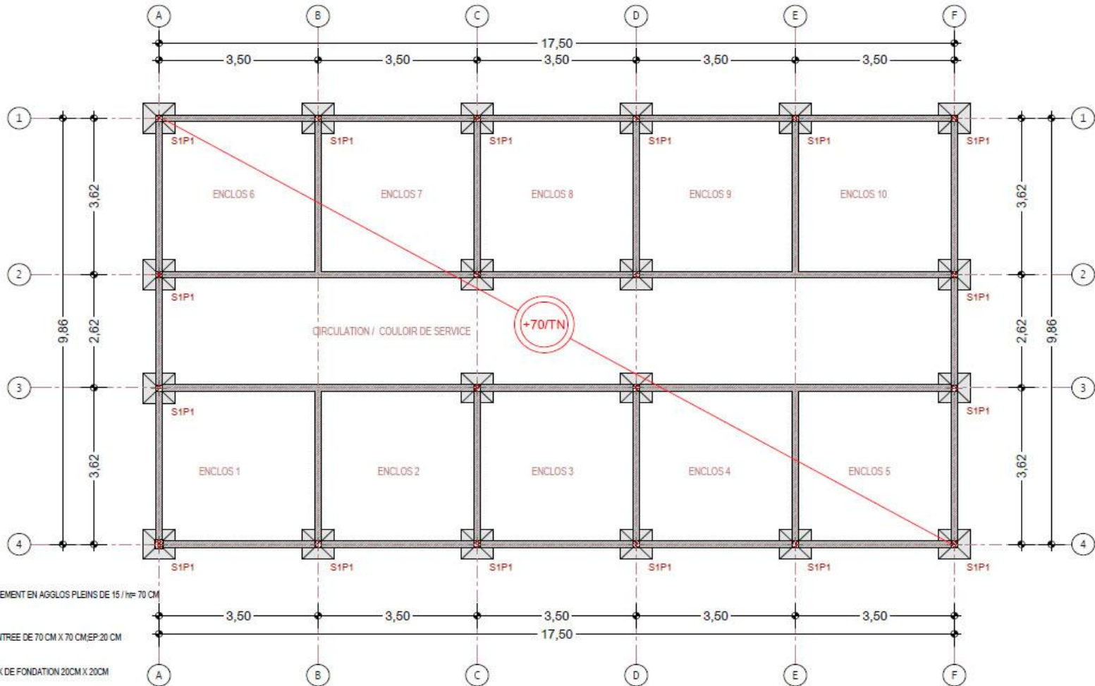
PLAN TYPE D'IMPLANTATION ET DE FONDATION / ETABLE CAPRINS ET OVINS
