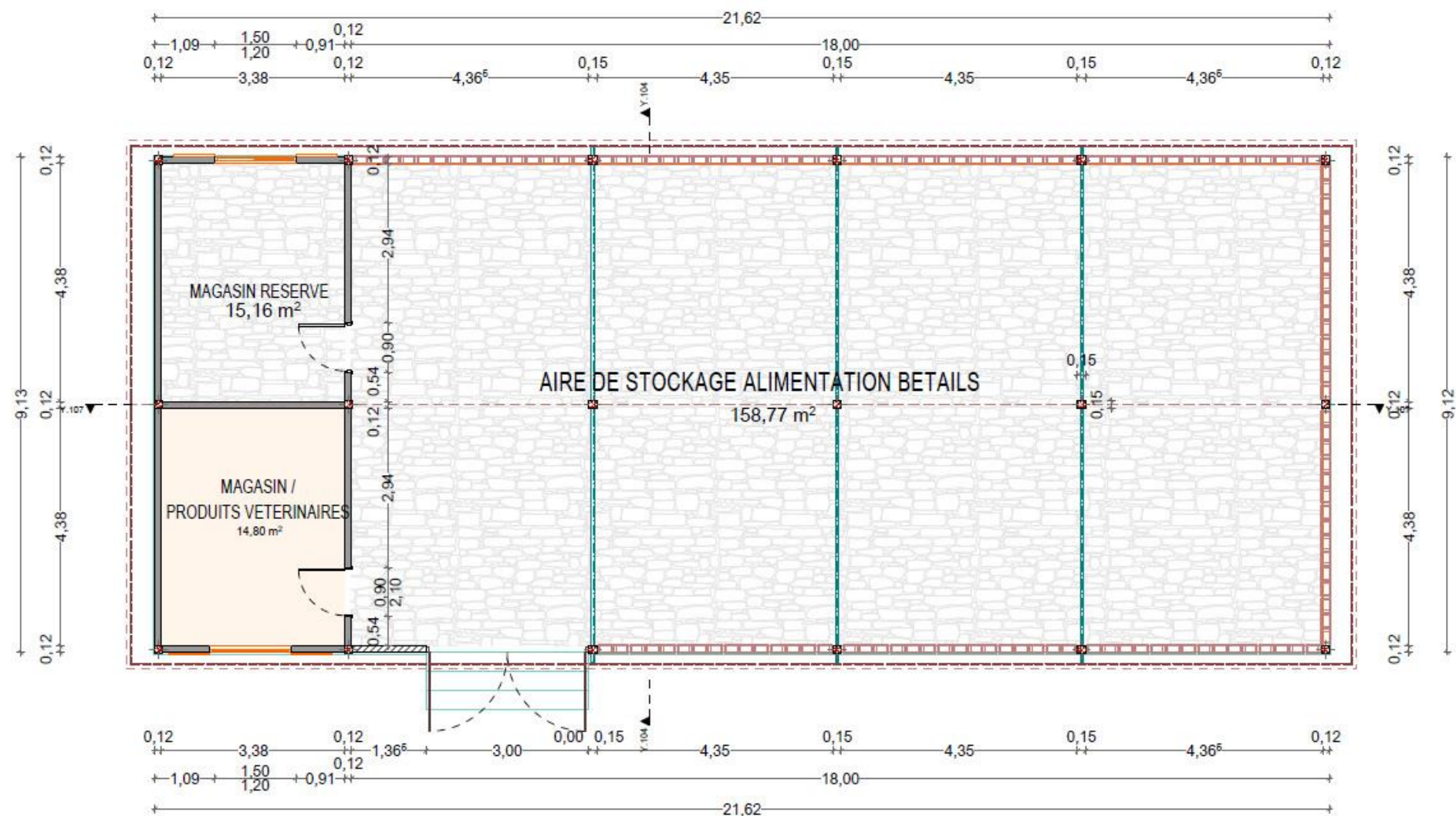
VUE EN PLAN COTE MAGASIN DE STOCKAGE ALIMENTATION BETAILS
